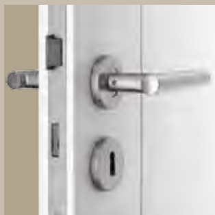
Dózický zámok trieda I, manžeta z niklového striebra (sériovo)
